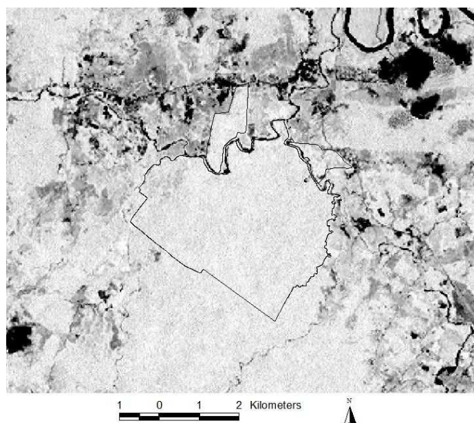
Figure 3. Estimated ENT image for La Selva Biological Station. The brighter the area, the higher the ENT. Figura 3. Imagem estimada ENT para Estação Biológica La Selva. Quanto mais clara fora área, maior do valor de ENT.
